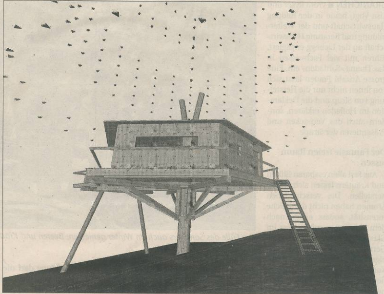
Das Baumhaus wird um den Eichenstamm gebaut, ohne dass Verbindungsmittel in den Baum montiert werden. Die Punkte deuten die Baumkrone an. (Bilder zVg)
